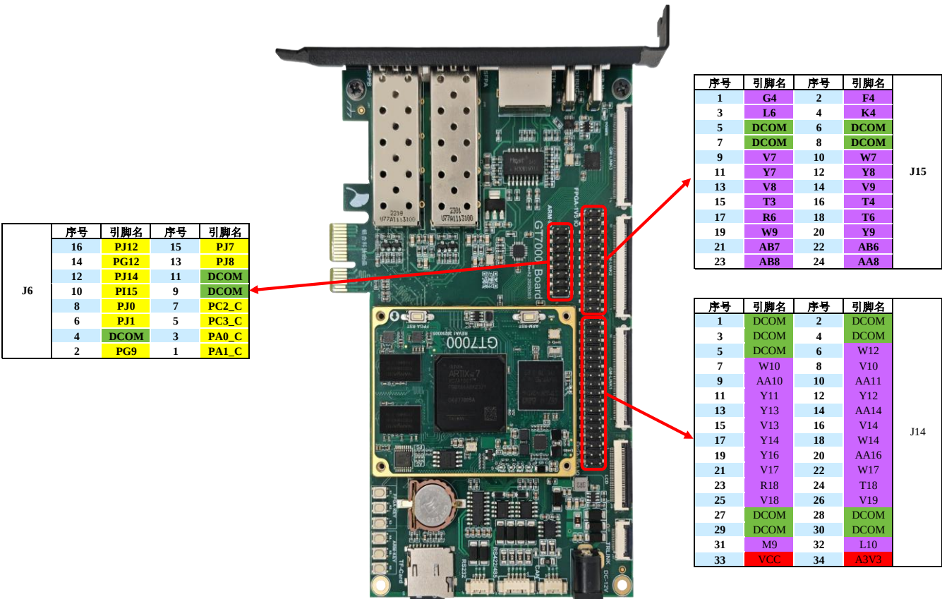
GT7000底板扩展引脚图V1.0
